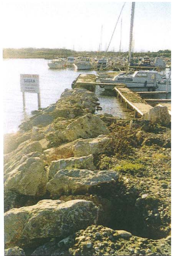
Enrochements de l'enracinement de la digue nord déplacés
