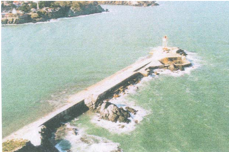
Digue du môle abri
