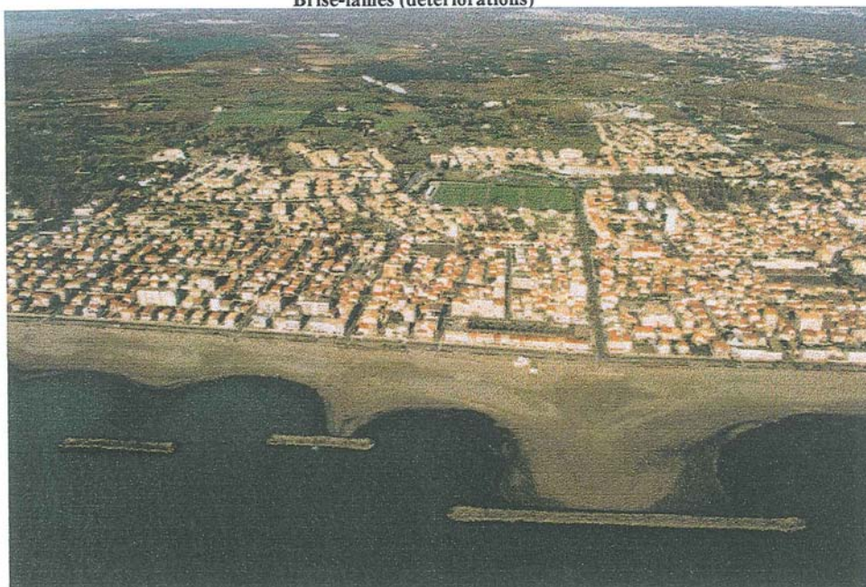
Brise-lames (détériorations)
